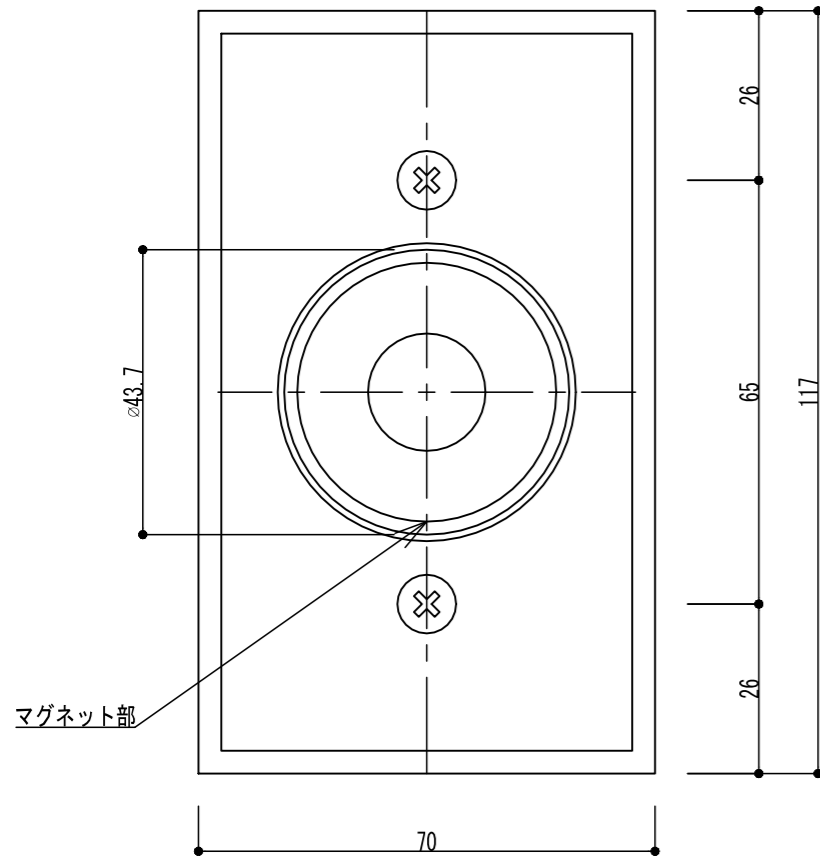
SEM7840 / 7850 << 背面図 >>
