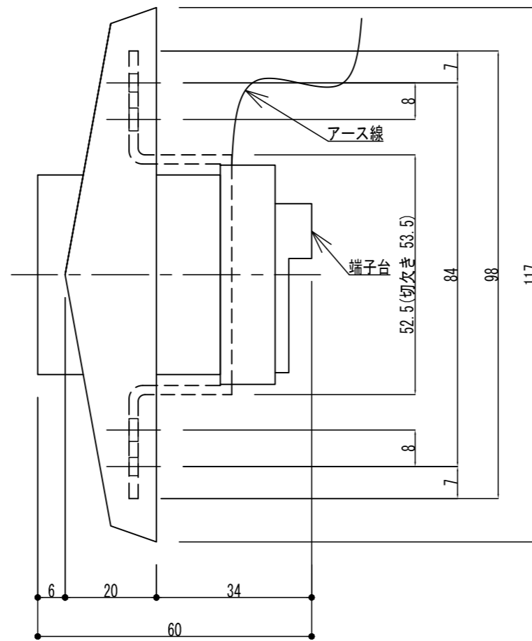
SEM7840 / 7850 << 側面図 >>
