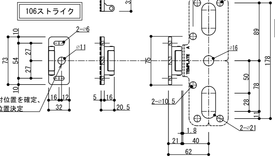
1100 ヘッド切欠テンプレート
