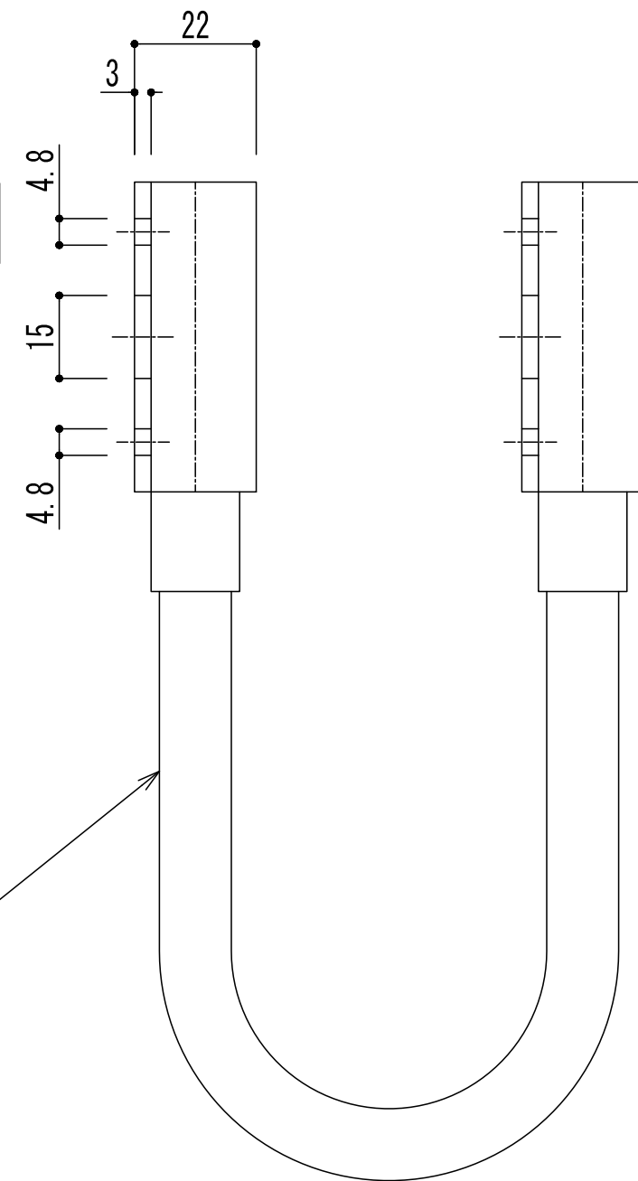
右側面図
