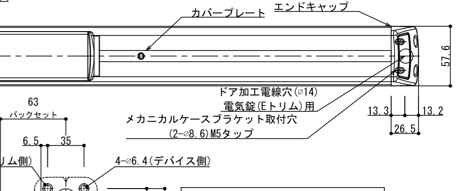
F1100 ヘッド切欠テンプレート
