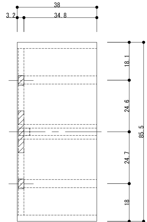
断面図
