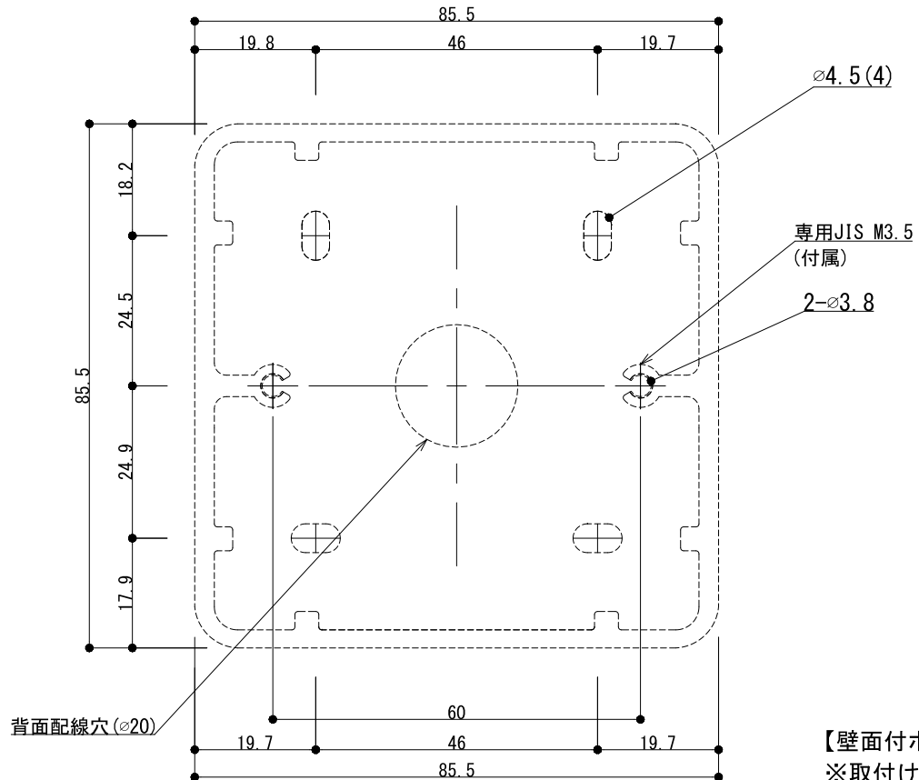
正面図
