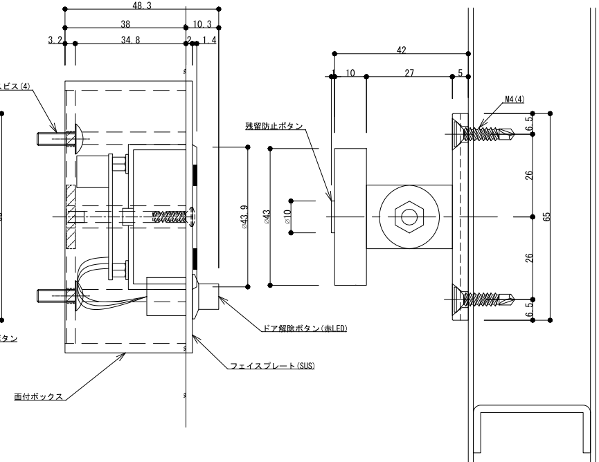
収まり 側面図
