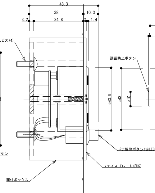
収まり 側面図
