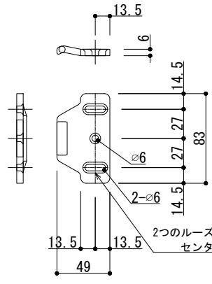
136R(両開用)ストライク
