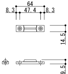
224ボトムストライク
