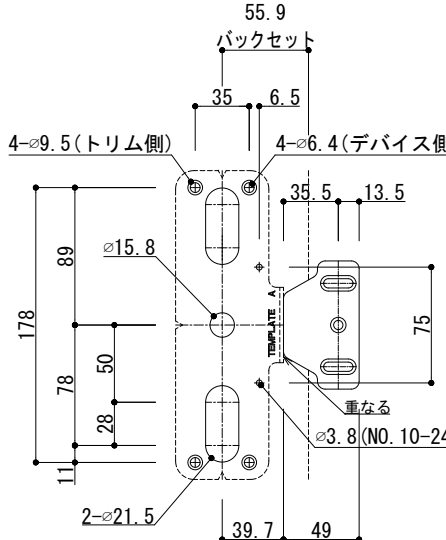
1100 ヘッド切欠テンプレート
