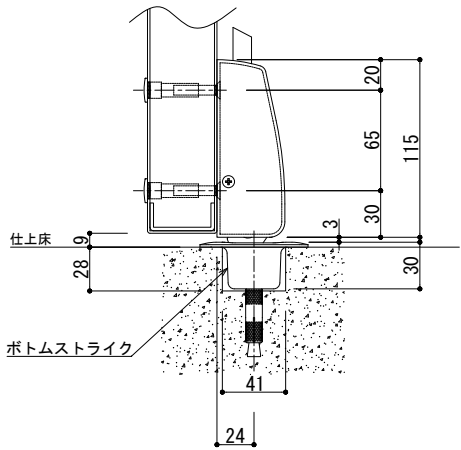
224ボトムストライク
