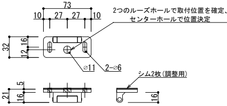
106 トップストライク
