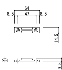
224 ボトムストライク
