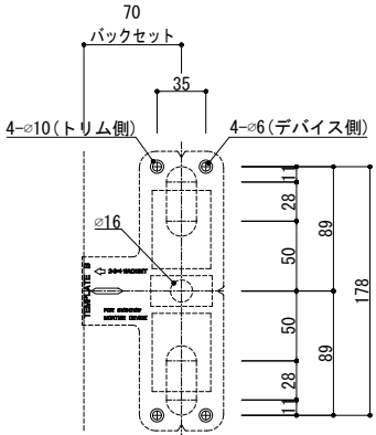
1200 ヘッド切欠テンプレート
