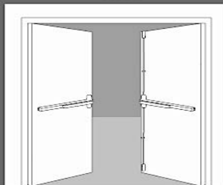
リムパニックバーと垂直ロッドパニックバー
